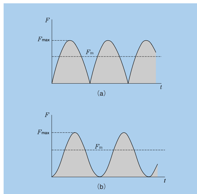
Fig. 4.11 Sinusoidal variable load
