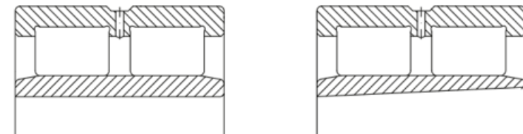
NNU TYPE
